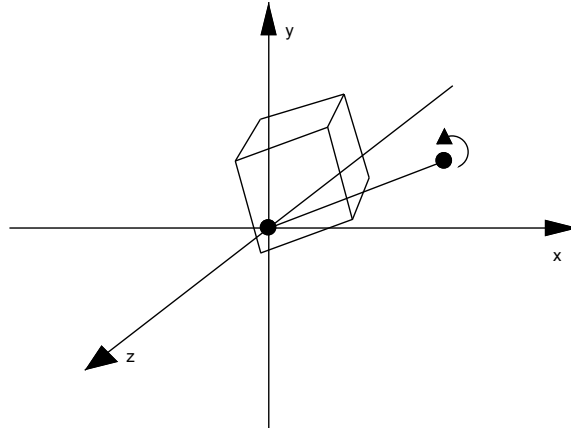
Rys 3.1 Sześcián obrócony o 90 stopni wokół wektora o współrzędnych [1,1,1].
