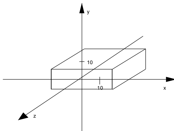
Rys 3.3 "Rozciągnięty" sześcián
