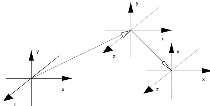
Rys. 4.3 Interpretacja przekształceń przestrzennych jako ciąg transformacji lokalnego układu współrzędnych
